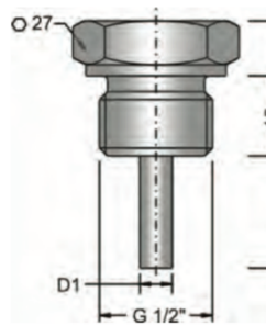
G 1/2" ISO 228-1
